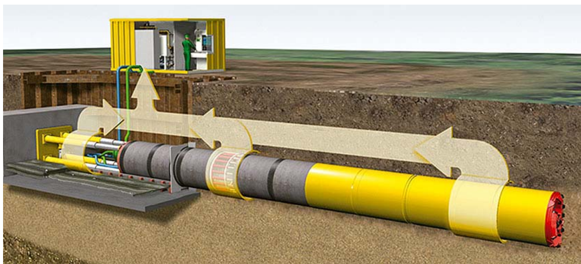
Figura 4: Esquema metodología constructiva pipe – jacking
